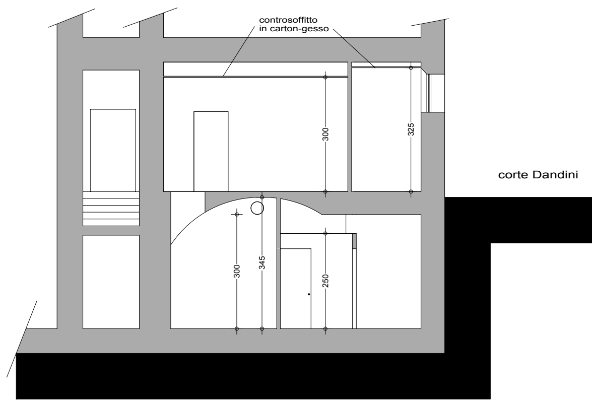
SEZIONE a-a
